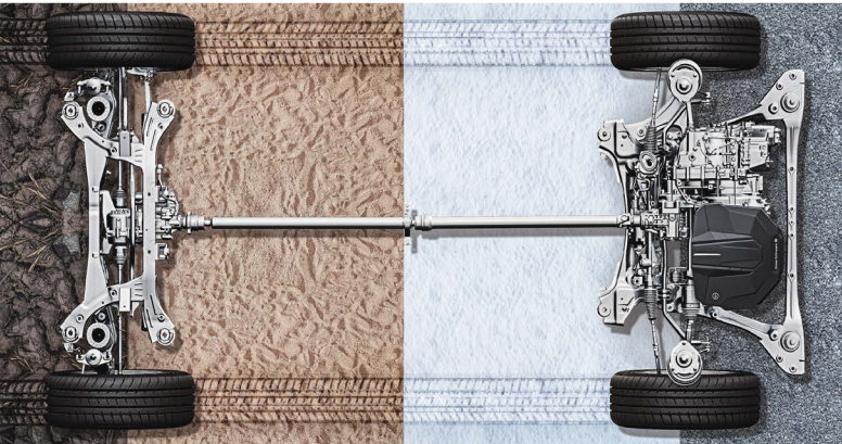
Torque Vectoring AWD
